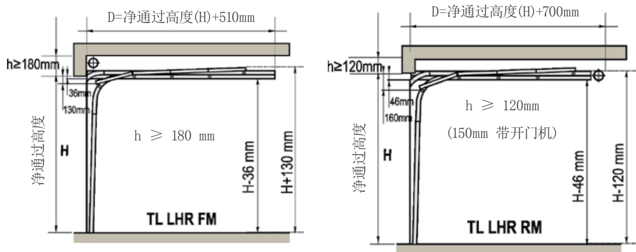
TL/LHR-FM 低顶部高度, 双轨道, 前方安装弹簧组件
